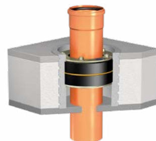
Variante: Curaflex® 3000 und Curaflex® C en tant que passage de dalles
